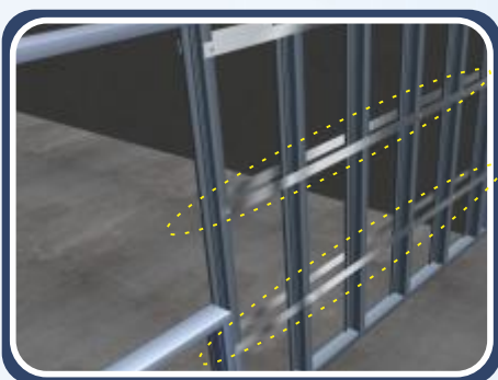
Fita de Contraventamento - Aplicação
